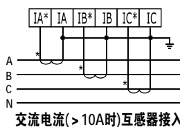
交流电流(>10A时)互感器接入
