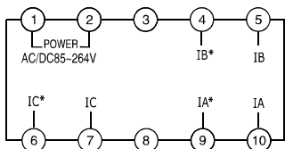
交流电流(≤10A)直接接入
