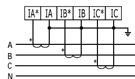
交流电流(>10A)互感器接入
