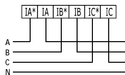
交流电流(≤10A)直接接入
